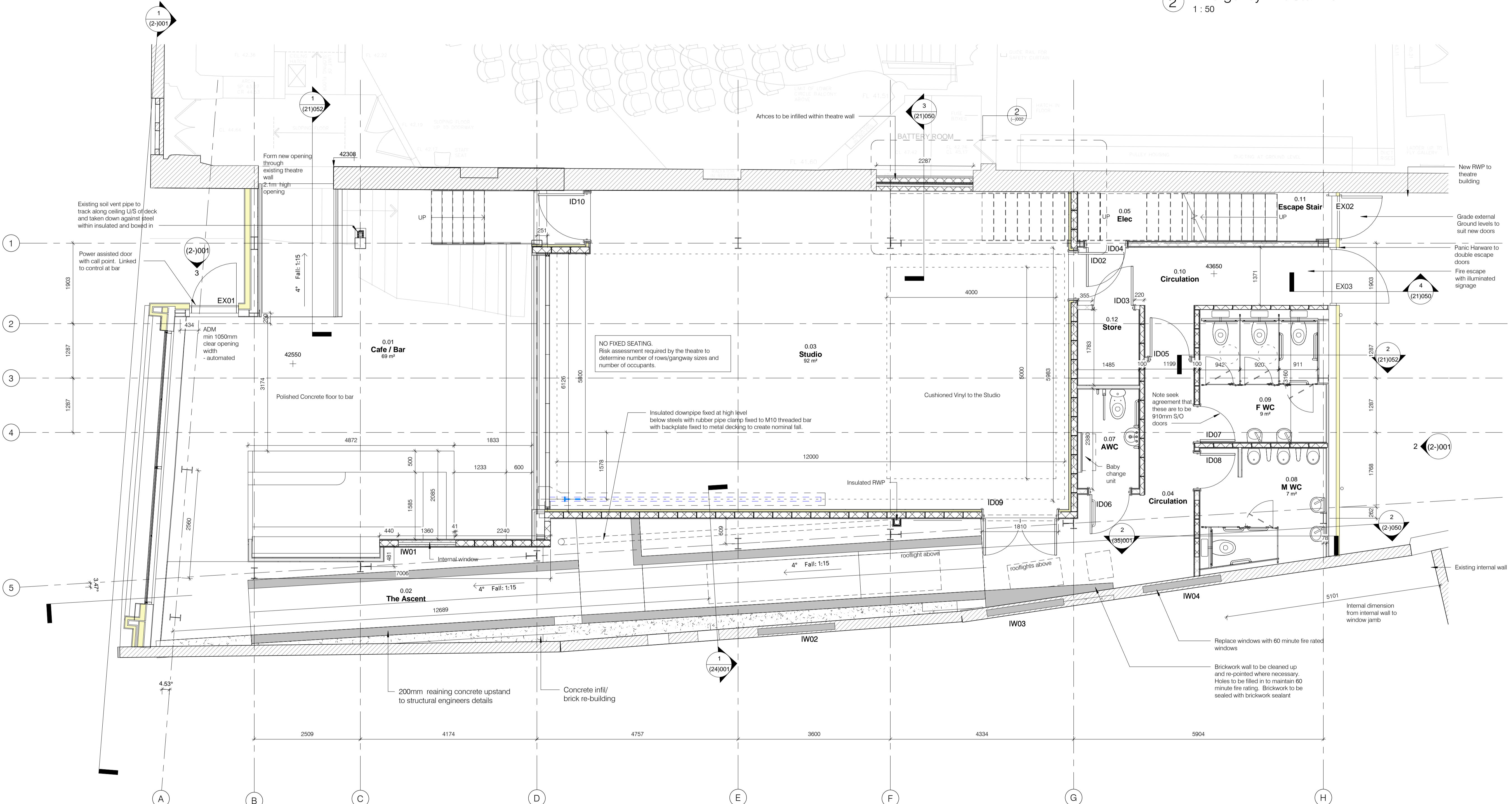
1 Level 0 GA 1 : 50
